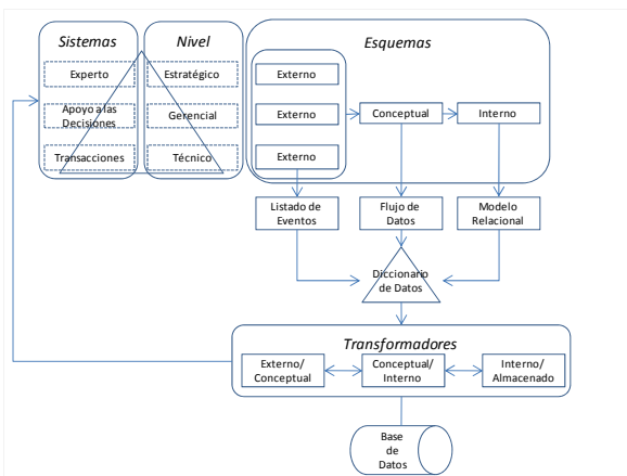
Figura 3 Sistema de Gestión de la Información
